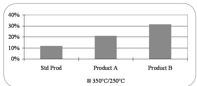
Fig. 4 Hot Die Adhesion Index. Indice di adesione a caldo dello stampo.
